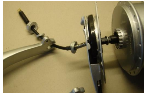
Foto 1.3 Rollerbrake
