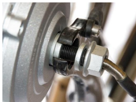
Foto 1.1 Velgrem
