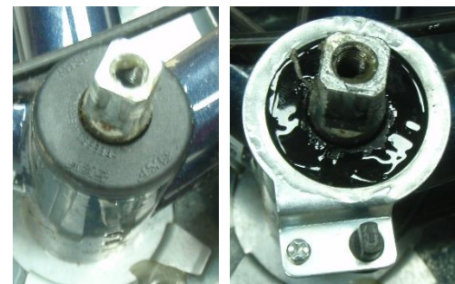
Foto 3.2: Geperste lagercup
